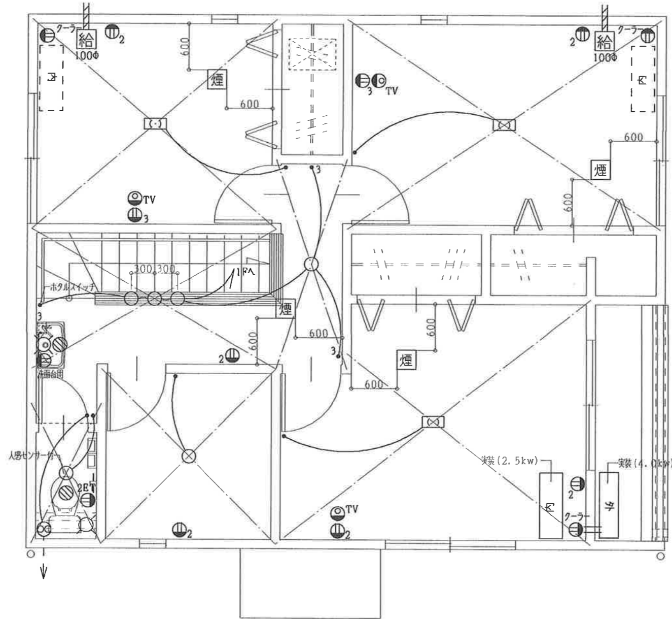
2階電気設備図
